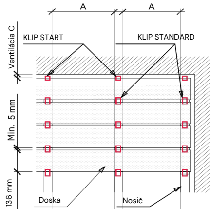
Obr. 4 Minimálne špáry medzi doskami a medzi doskami a pevným múrom
